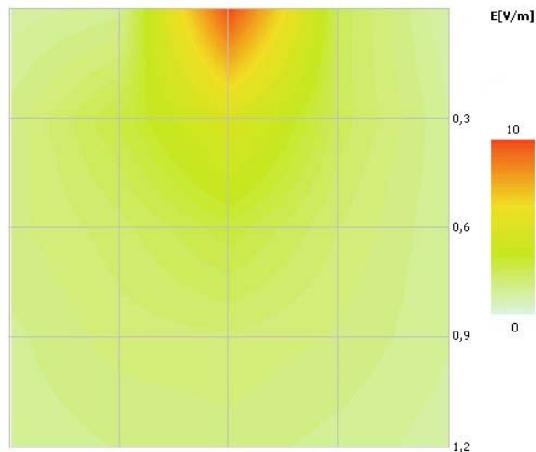
Rys. 14. Natężenie pola EM za bramką RFID bez absorberów.
