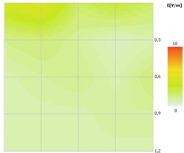
Rys. 15. Natężenie pola EM za bramką RFID z absorberami.
