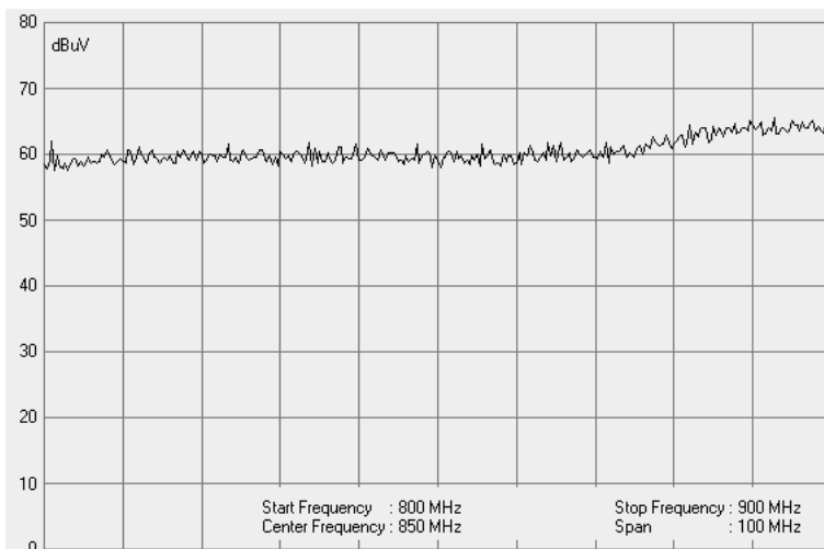
Rys. 11. Tłumienność absorbera C
