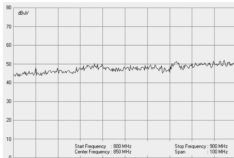
Rys. 10. Tłumienność absorbera B
