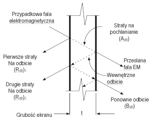
Rys. 1. Straty na przewodzącym ekranie z ciała stałego [1]
