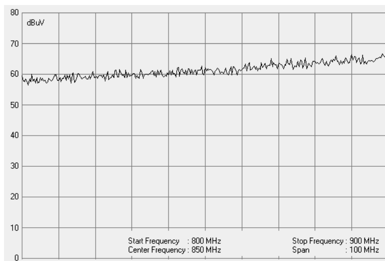
Rys. 8. Poziom zaburzenia w układzie bez absorberów
