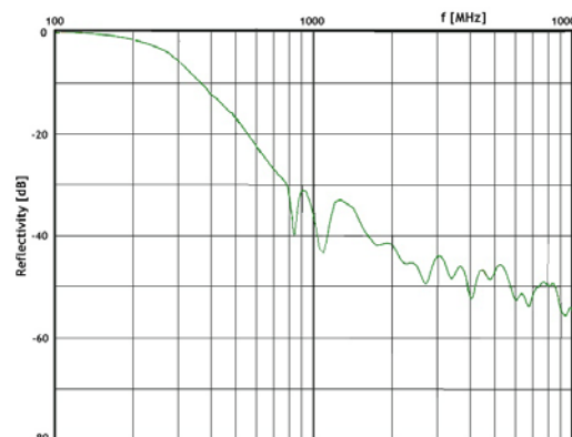
Rys. 3. Współczynnik odbicia absorbera A.
