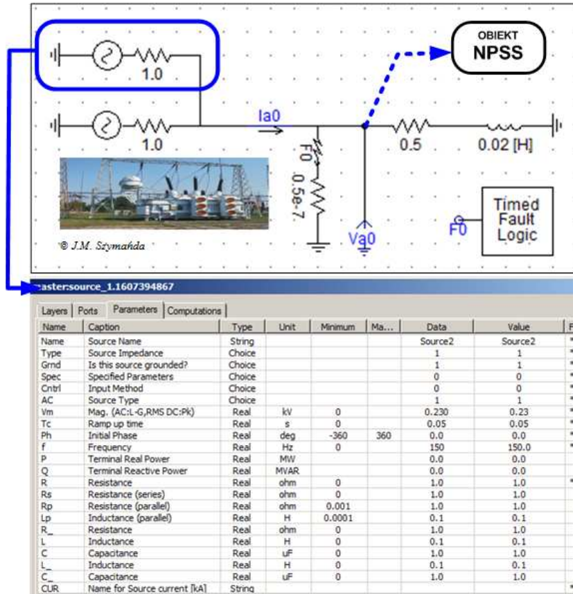
Rys.7. Wybrany wariant indywidualnego bloku z przykładowymi parametrami elektrycznymi obiektu; „Timed Fault Logic” – programator zdarzeń czasowych dla zdefiniowanych lokalnych awarii (np.zwarcia)
