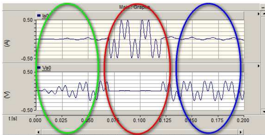
Rys.8. Obserwacje charakterystycznych przebiegów czasowych obiektu w węzle NPSS; kolorami oznaczono cechy obiektu dla stanów: niestabilnych (zielony), awarii-zwarcia (czerwony), ustalonych (niebieski)
