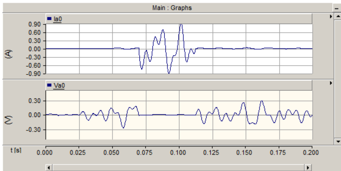
Rys.10. Obserwacje charakterystycznych przebiegów czasowych obiektu w węzle NPSLogistics A
