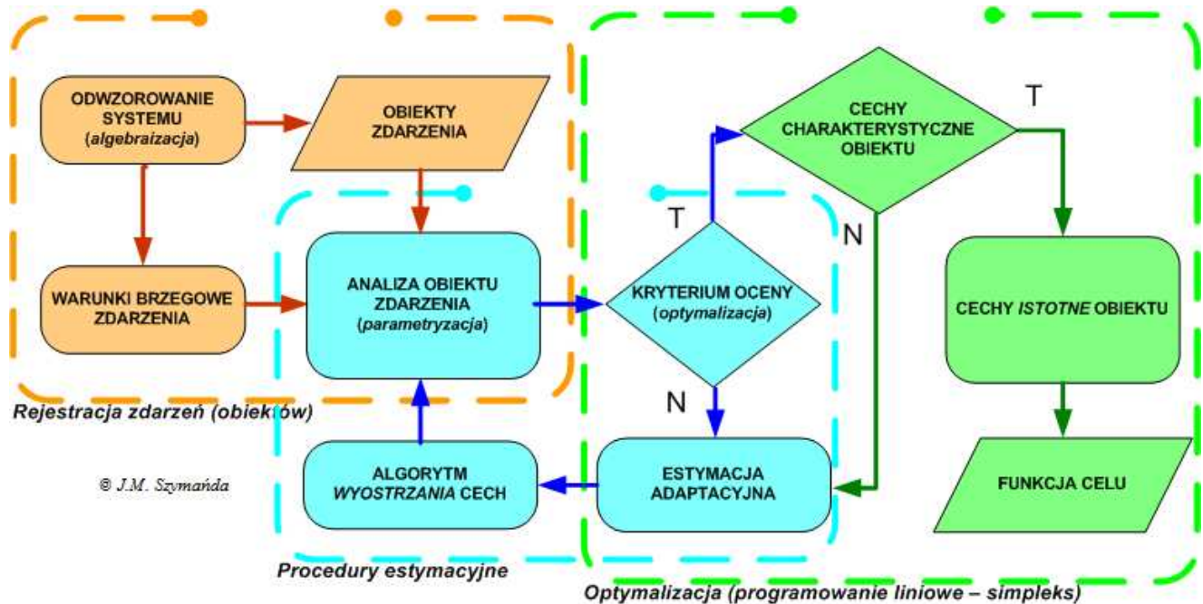
Rys.1. Wariant diagramu przepływu informacji w procedurach wyznaczania istotnych cech obiektu
