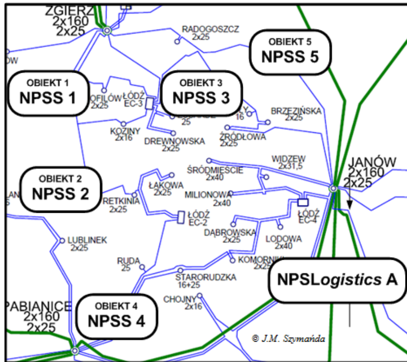
Rys.6. Poglądowy schemat sieci elektroenergetycznej z naniesionymi węzłami NPSS oraz NPSLogistics
