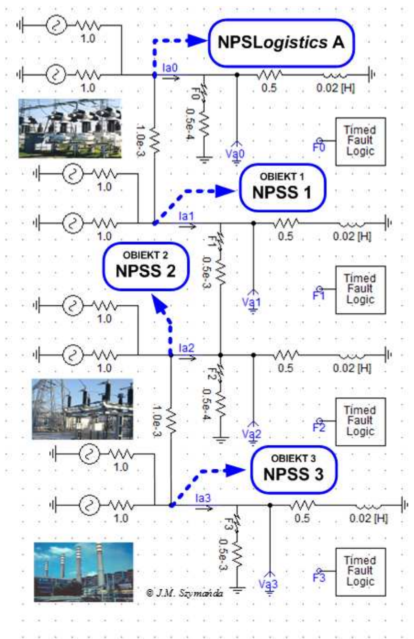
Rys.9. Przykładowy schemat elektryczny modelu propagacji zaburzeń w sieci elektroenergetycznej, „Timed Fault Logic” – programator zdarzeń czasowych dla zdefiniowanych lokalnych awarii
