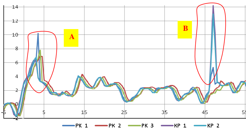
Rys. 2. Wykres szerokości toru zasadniczego rozjazdu Nr 1: PK – początek, koniec, KP – koniec początku, 1 – numer pomiaru
