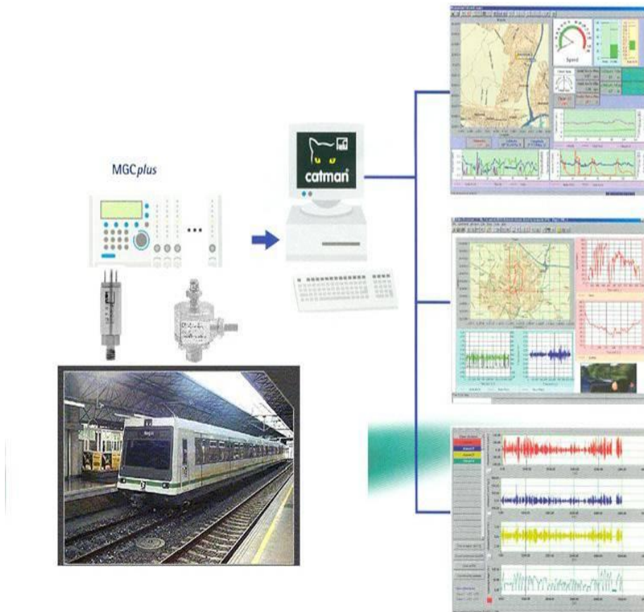
Rys.5 System pomiarowy do oceny bezpieczeństwa i komfortu jazdy [4,5]
