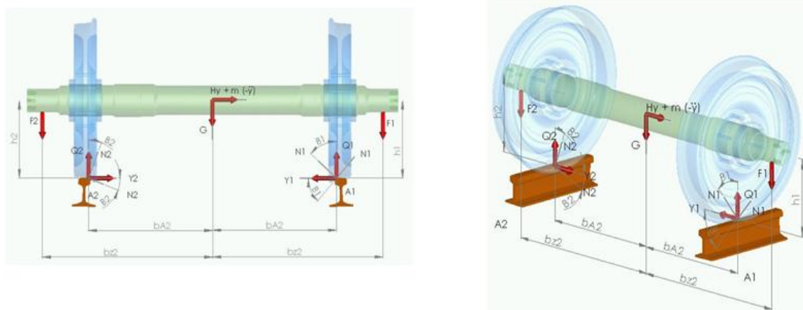
Rys.3 Rozkład sił zestawu oś-koło na szynę
