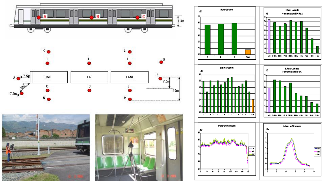
Rys.4 Pomiar poziomu hałasu wewnątrz i na zewnątrz pojazdu kolejowego
