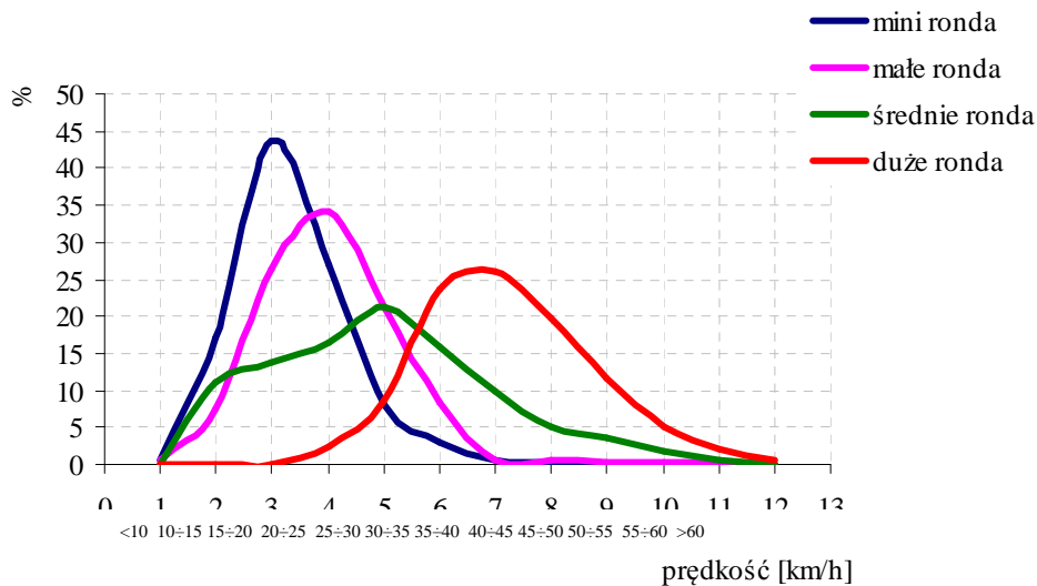
Rys. 3. Rozkład częstości występowania poszczególnych prędkości pojazdów na skrzyżowaniach typu rondo
