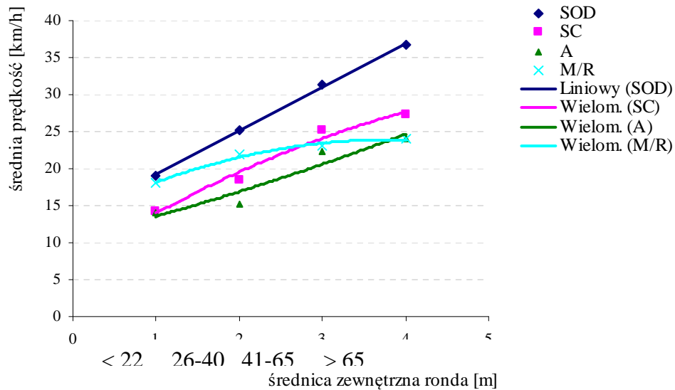
Rys. 5. Zależność średniej prędkości z jaką poruszają się pojazdy po rondach od średnicy zewnętrznej ronda, gdzie: SOD – samochody osobowe i dostawcze, SC – samochody ciężarowe, A – autobusy, M/R – motocykle i rowery
