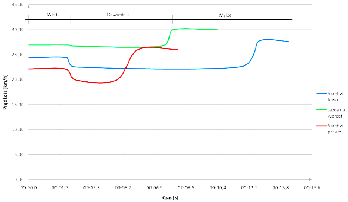
Rys. 6. Prędkości samochodów osobowych i dostawczych podczas przejazdu przez rondo (I typ linii prędkości pojazdów na rondzie)
