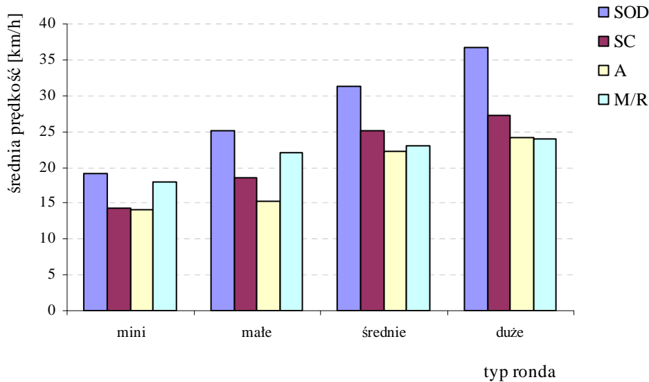
Rys. 4. Średnie prędkości przejazdu poszczególnych grup rodzajowych pojazdów po skrzyżowaniach typu rondo gdzie: SOD – samochody osobowe i dostawcze, SC – samochody ciężarowe, A – autobusy, M/R – motocykle i rowery.
