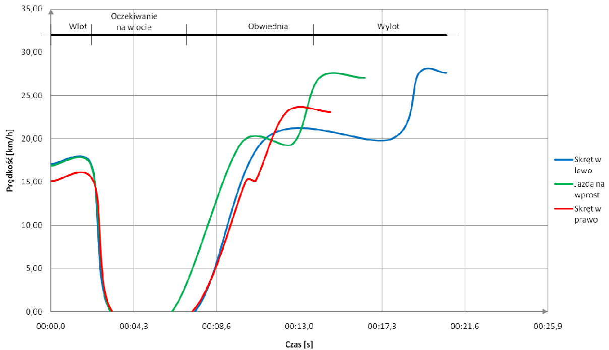
Rys. 7. Prędkości samochodów osobowych i dostawczych podczas przejazdu przez rondo (II typ linii prędkości pojazdów na rondzie)
