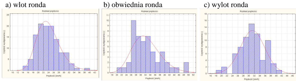
Rys. 2. Empiryczne rozkłady prędkości pojazdów z naniesionymi rozkładami teoretycznymi dla a) wlotu ronda, b) obwiedni ronda, c) wylotu ronda
