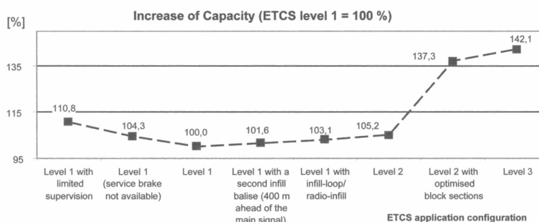
Rys. 13. Obliczona przepustowość dla przypadku linii konwencjonalnych
