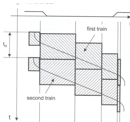
Rys. 6. Optymalizacja sekcjonowania blokady dla ETCS poziom 2
