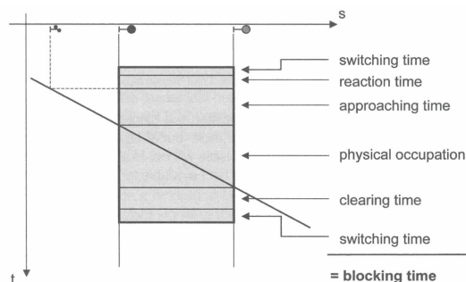
Rys. 1. Składniki czasu blokowania
