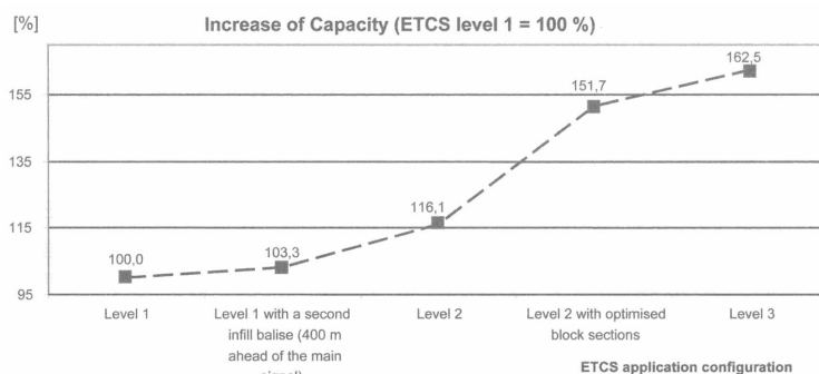
Rys. 11. Obliczona przepustowość dla przypadku linii dużych prędkości
