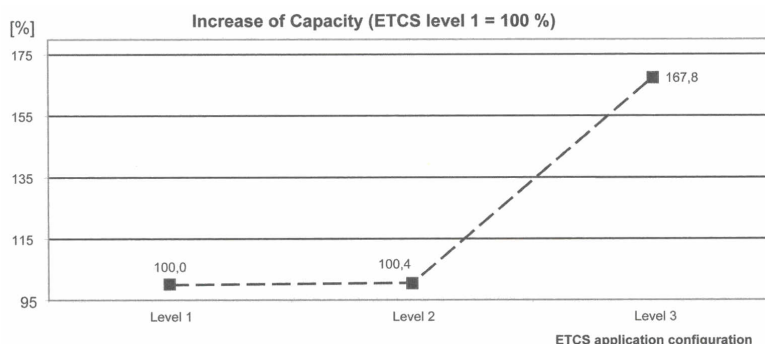
Rys. 15. Obliczona przepustowość dla przypadku linii regionalnych
