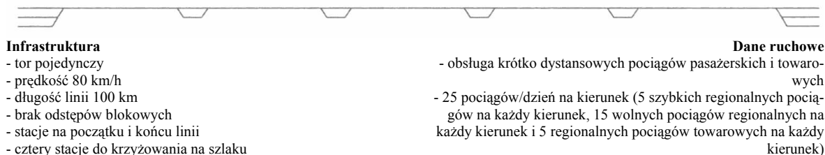
Rys. 14. Układ torowy i schemat ruchowy dla przypadku linii regionalnych
