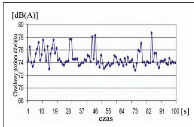
Rys. 10. Chwilowa wartość poziomu hałasu w trakcie postoju pojazdu – miejsce pomiarowe nr 6 dla pojazdu 3.
