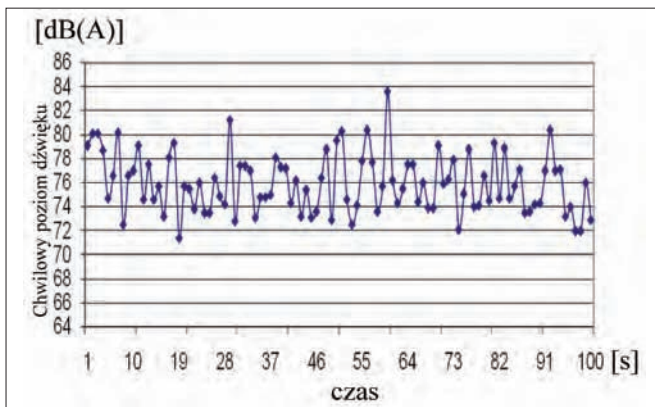
Rys. 8. Chwilowa wartość poziomu hałasu w trakcie postoju pojazdu – miejsce pomiarowe nr 1 dla pojazdu 3.
